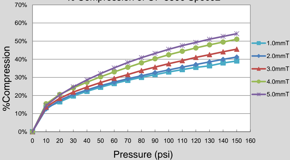
% Compression of OP 8500 Spec02
